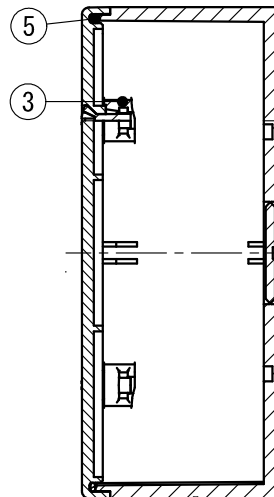
断面 A-A
